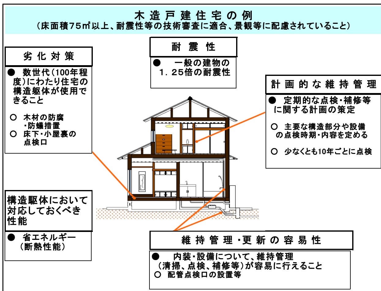
図 長期優良住宅のイメージ
